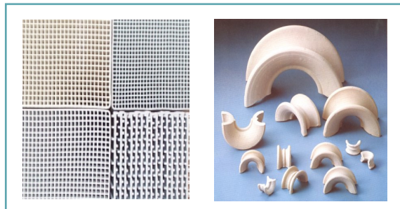
Figura 2. Diferentes medios cerámicos de intercambio de calor utilizado e los sistemas de oxidación térmica regenerativa
