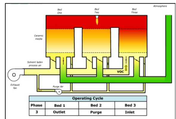
Figura 4. Funcionamiento de un RTO de tres lechos.
